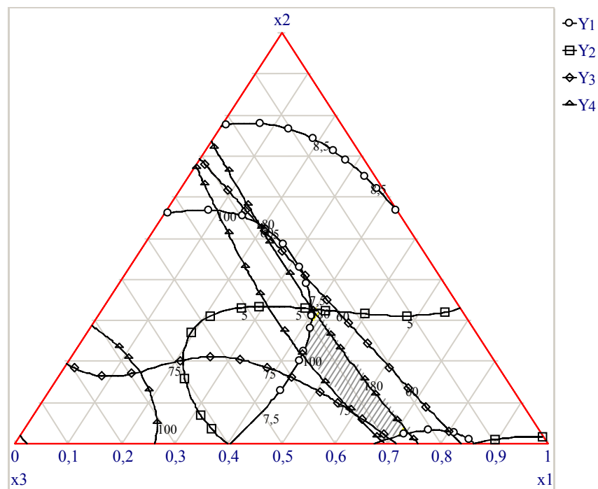
Рис. 4.14. Компромісна область складу ВДФ та експлуатаційних властивостей покриттів з них
