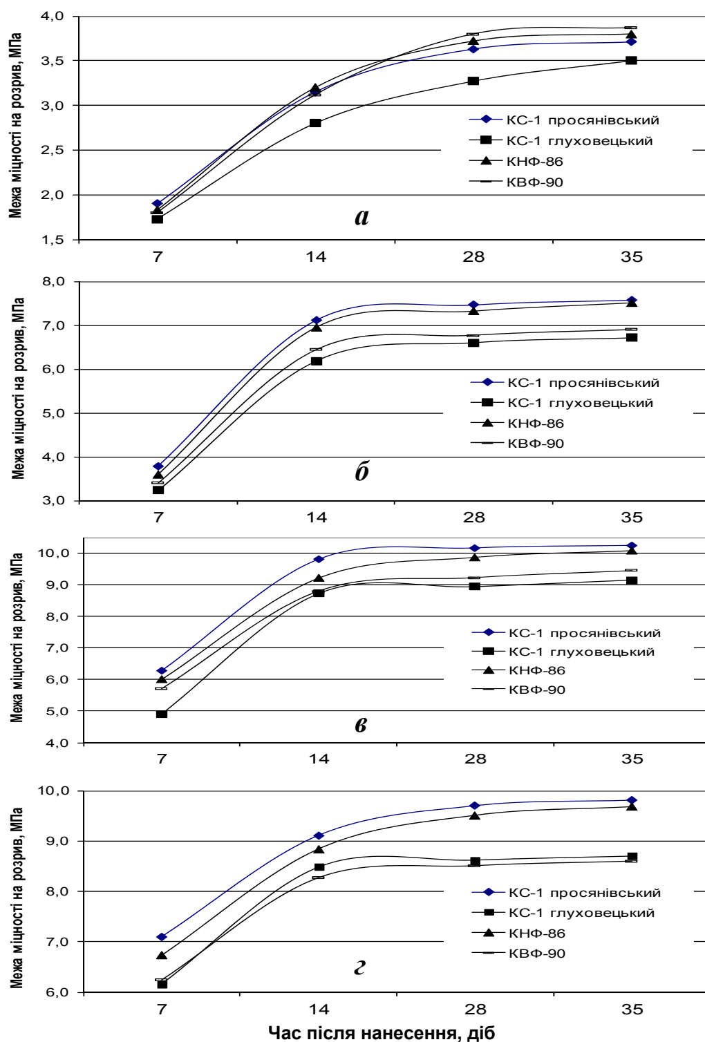
Рис. 4.3. Залежність межі міцності на розрив плівок з наповнених каолінами ВДФ від часу після нанесення та ОКН: a – 30 об. %; б – 40 об. %; в – 50 об. %; г – 60 об. %.
