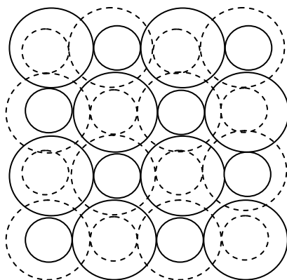
Рис. 3.1. Схематичне зображення моделі пірамідального типу упакування карбонатних наповнювачів з частинок різного розміру
